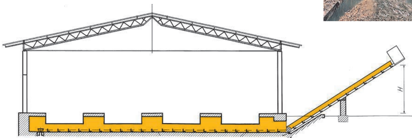
ダブルチェーンコンベア DOUBLE-CHAIN CONVEYOR
